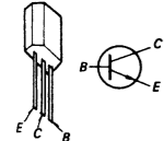
Q308 (408): 2SC945
